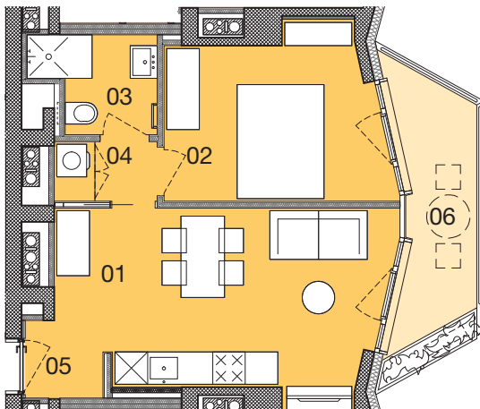
tloris stanovanja
