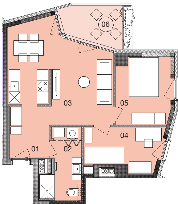
tloris stanovanja
