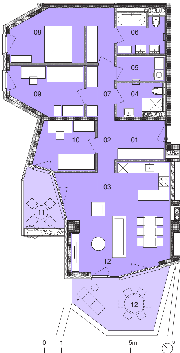
tloris stanovanja
