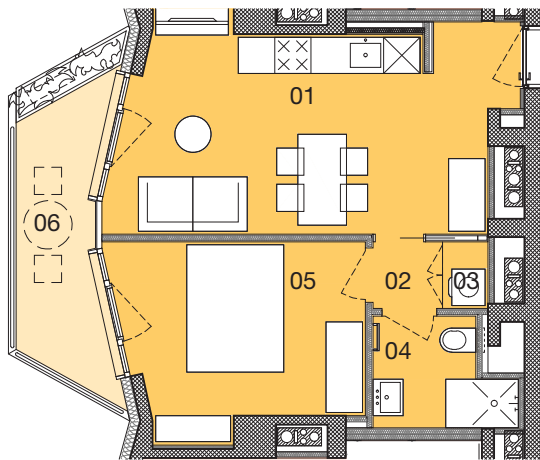
tloris stanovanja
